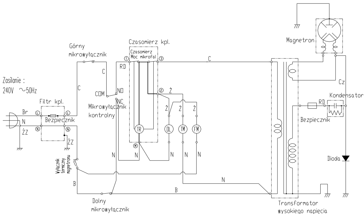
Schemat podłączeń przewodów do mikrowyłączników i czasomierza.
