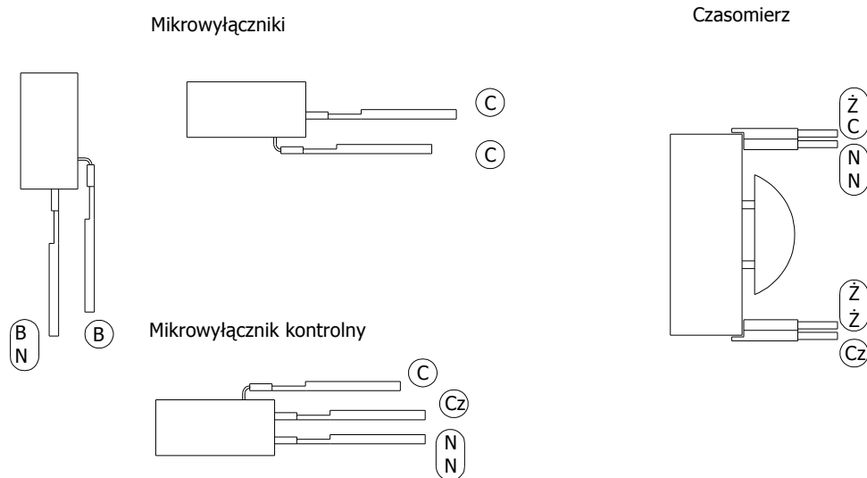
Schemat podłączeń przewodów do mikrowyłączników i czasomierza.
