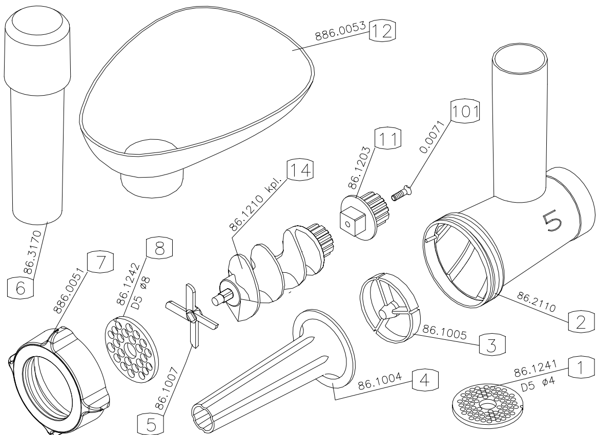
Rysunek części i podzespołów komory nr 5 (z nożykiem jednostronnym)
