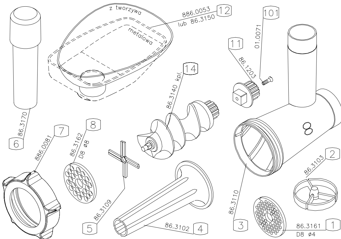
Rysunek części i podzespołów komory nr 8 (z nożykiem dwustronnym)
