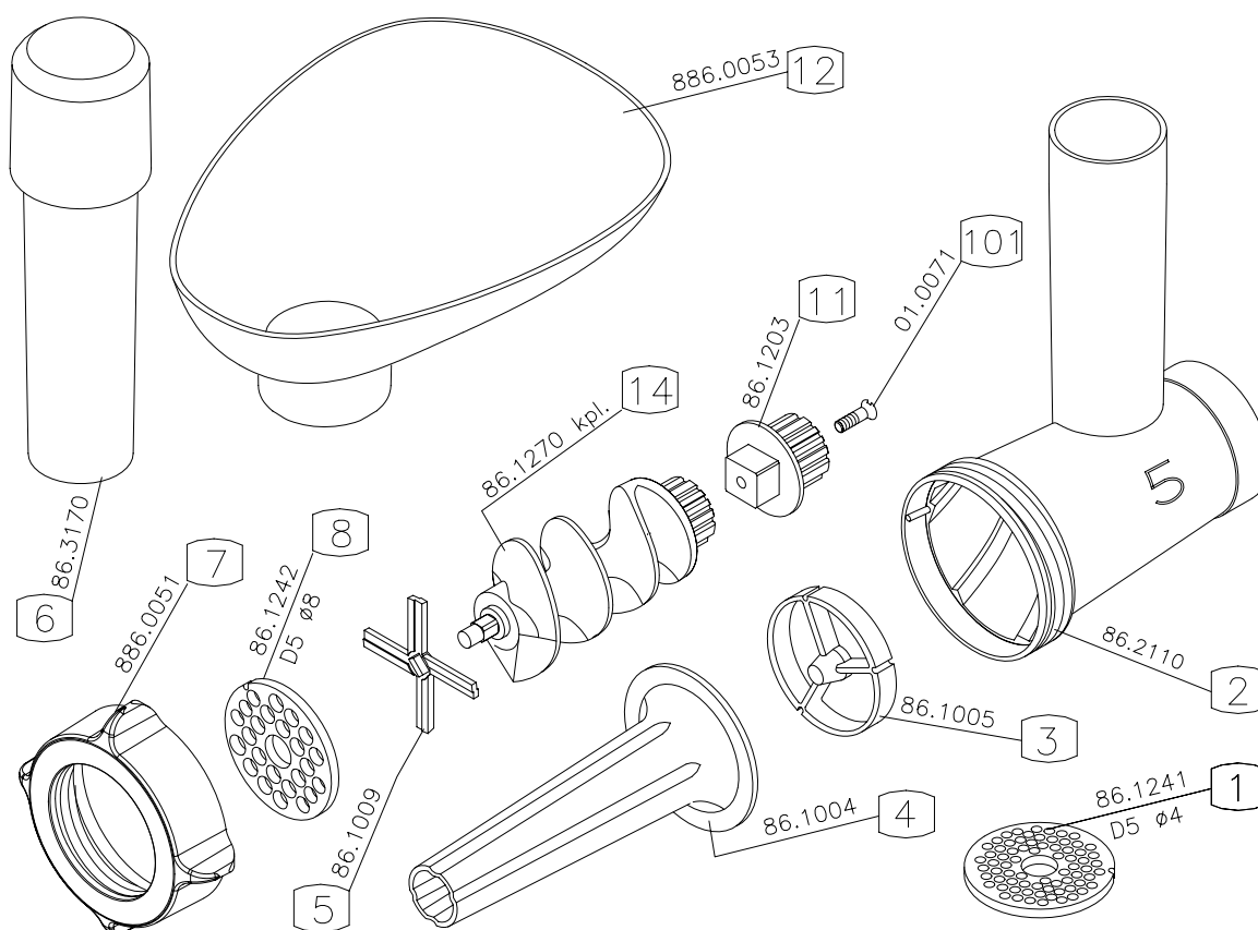
Rysunek części i podzespołów komory nr 5 (z nożykiem dwustronnym)
