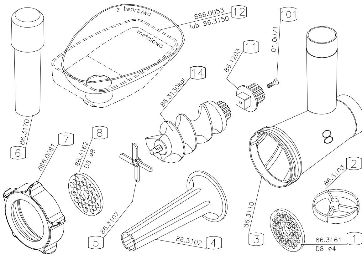
Rysunek części i podzespołów komory nr 8 (z nożykiem jednostronnym)
